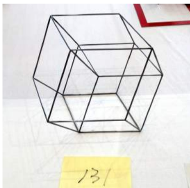
四つの平行四辺形 吉田 二郎 [京都府]
